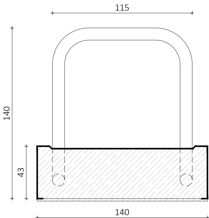
Tvöfaldir tengijárnabakkar Mkv. 1:2 Stærð bakka 43x140
