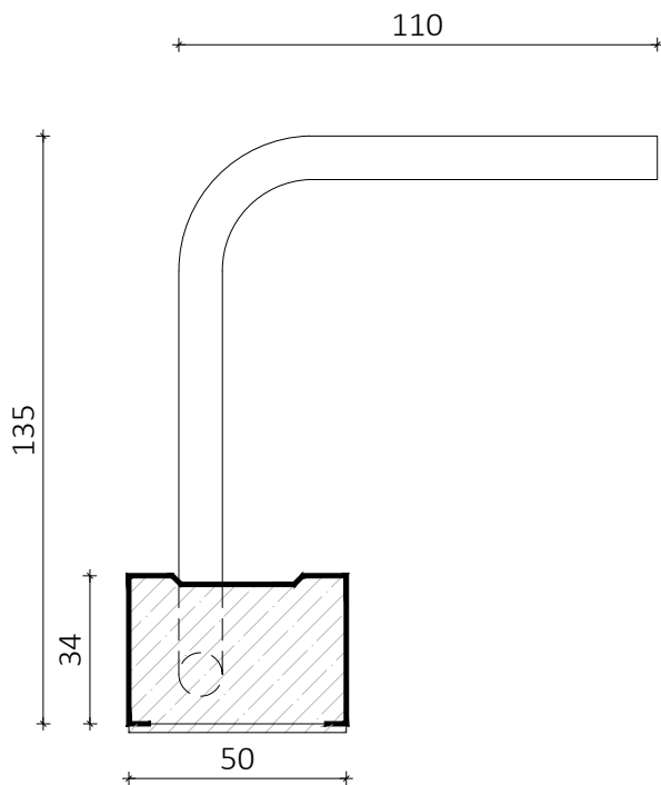
Einfaldir tengijárnabakkar Mkv. 1:2 Stærð bakka 34x50
