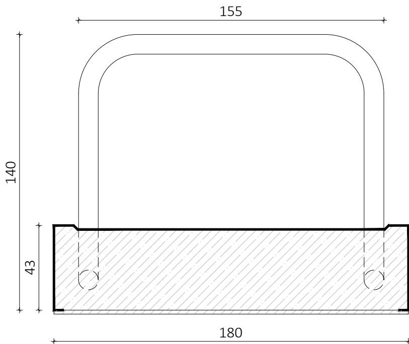
Tvöfaldir tengijárnabakkar Mkv. 1:2 Stærð bakka 43x180
