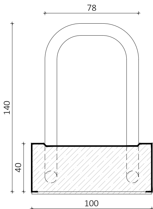
Tvöfaldir tengijárnabakkar Mkv. 1:2 Stærð bakka 40x100
